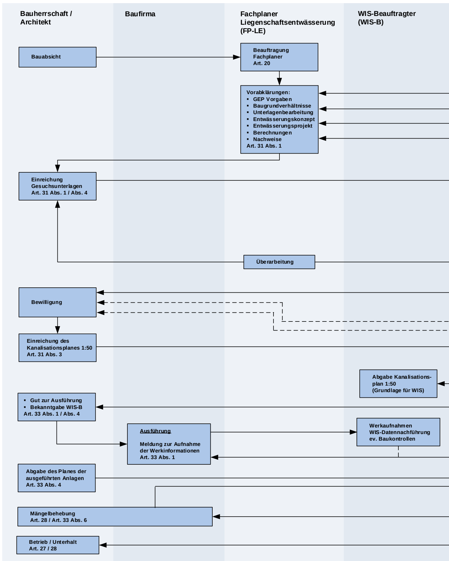
Abb. 19: Ablaufdiagramm Baugesuch Liegenschaftsentwässerung mit Verweis auf Artikel im Abwasserreglement
